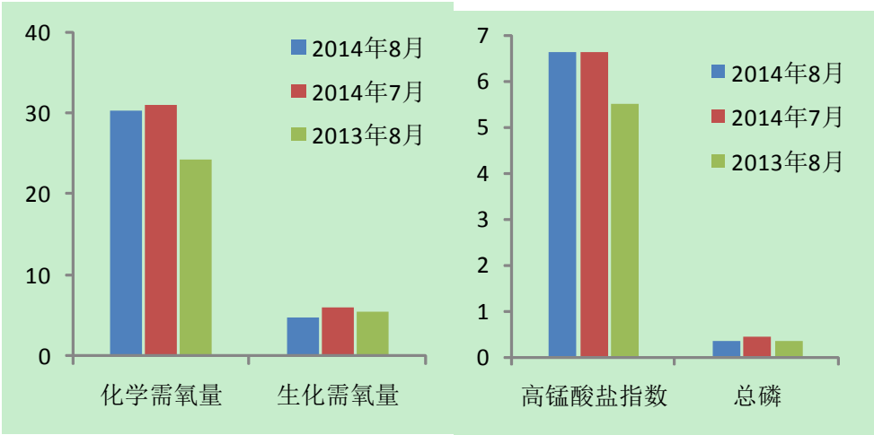
图2 河北省 2014 年 8 月河流主要污染物浓度变化情况
