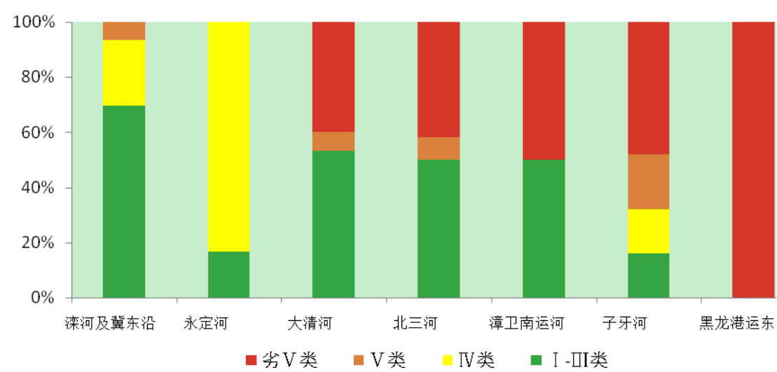
图3 河北省 2014 年 8 月七大水系水质状况
