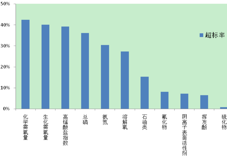
图 1 河北省 2014 年 8 月河流污染指标超标率统计
