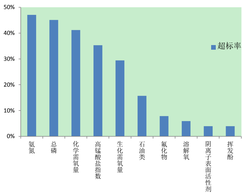
图 1 河北省 2015 年 2 月河流污染指标超标率统计
