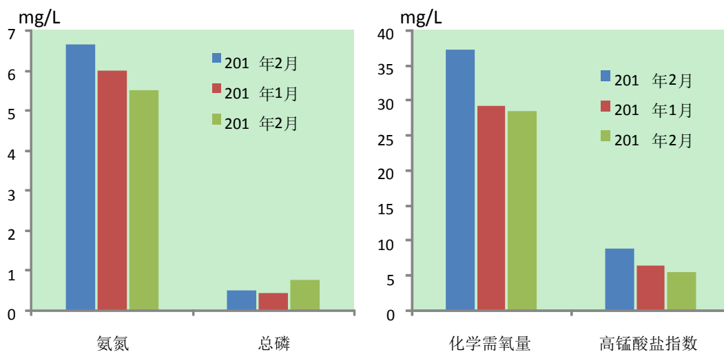
图2 河北省 2015 年 2 月河流主要污染物浓度变化情况
