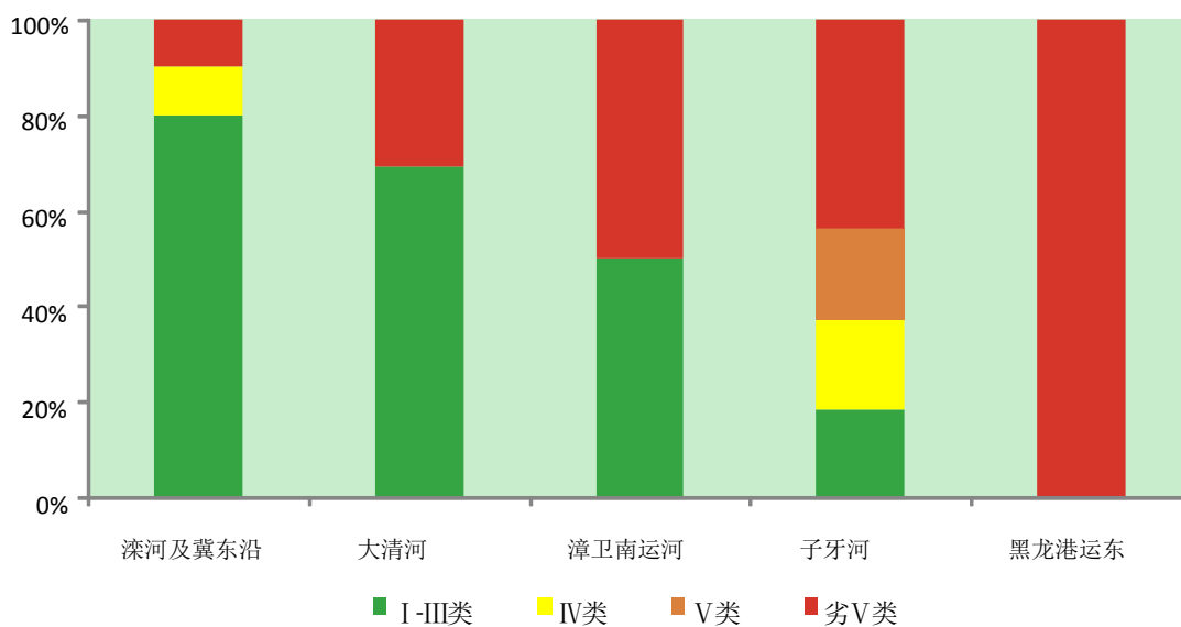
图3 河北省 2015 年 2 月七大水系水质状况
